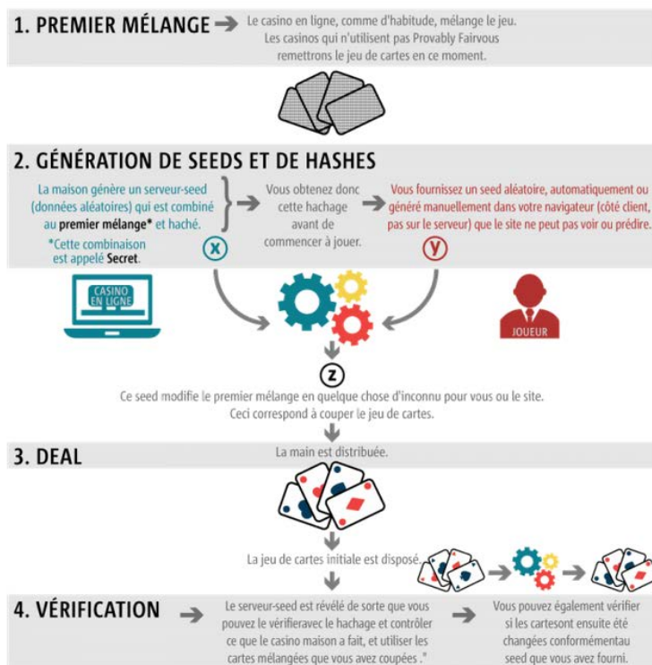
Figure 4 – Fonctionnement des jeux à équité prouvée
